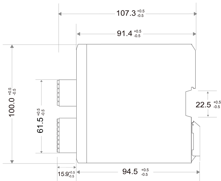
单位: mm
